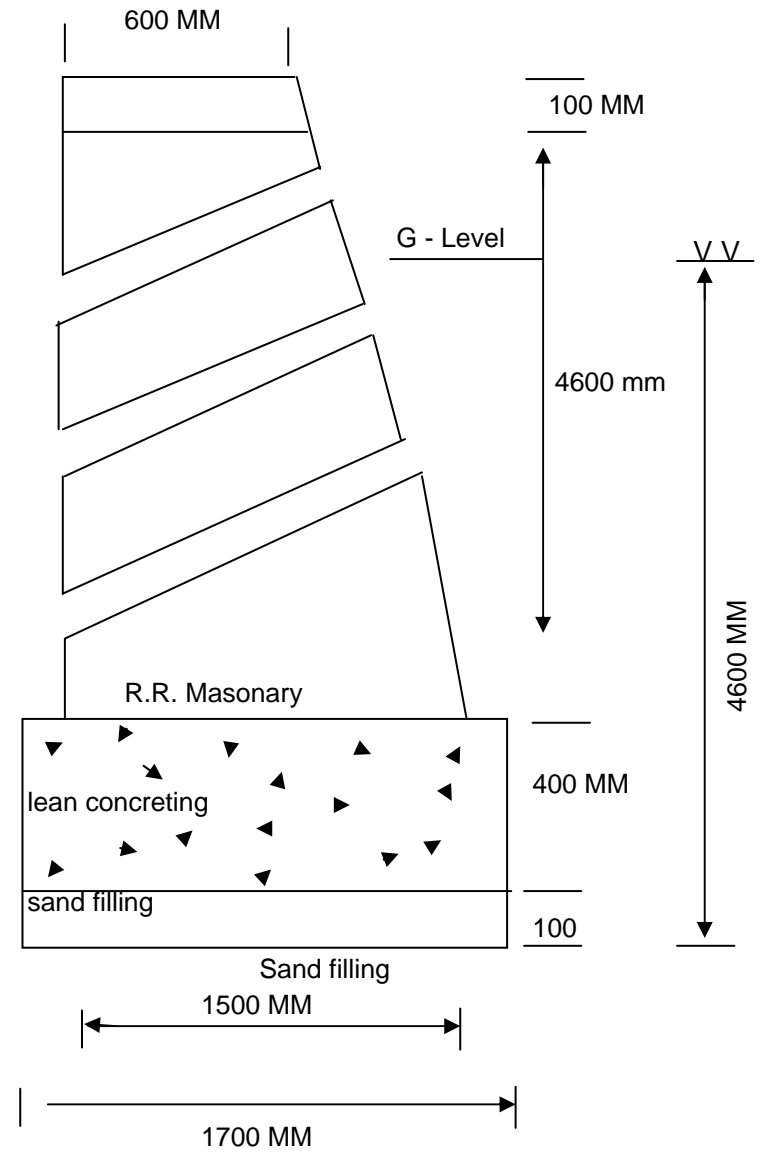
ELEVATION
